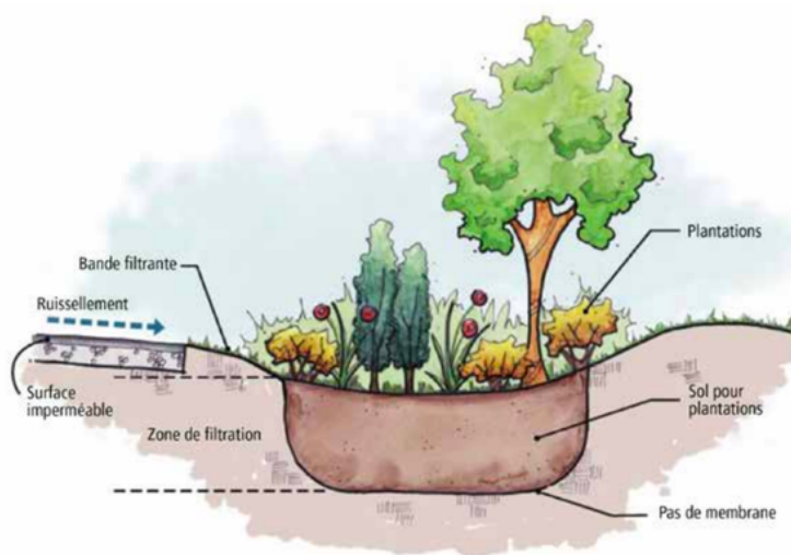
Figure 11.30 Section type sans drain (adapté de Hinman, 2005).
